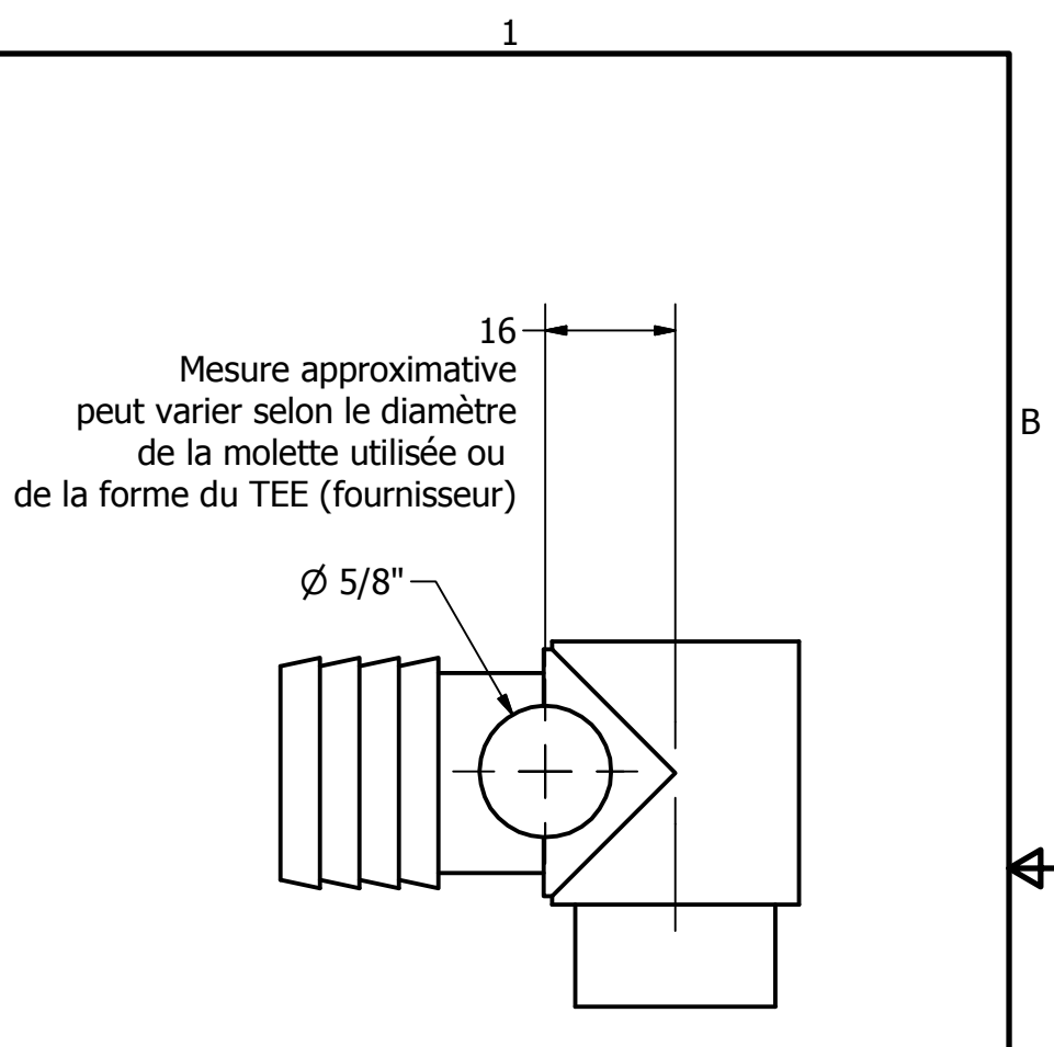
TEE à insertion en poly 1'' ECHELLE 1 : 1
